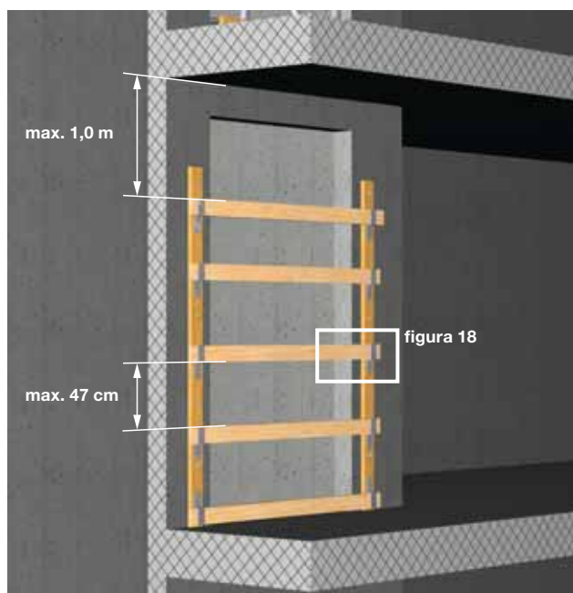
17 Apertura con protezione laterale sufficientemente alta.
