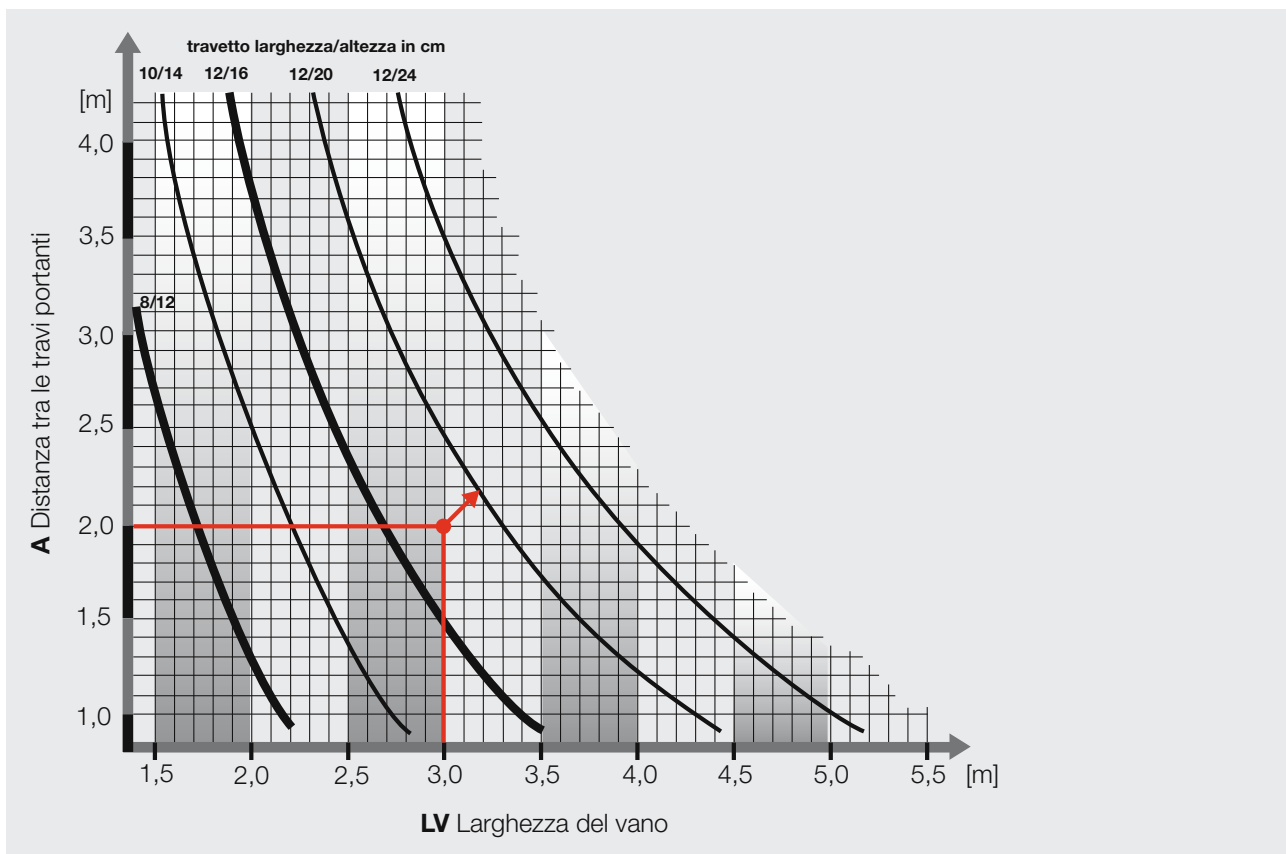
Diagramma 1: Diagramma per calcolare le dimensioni dei travetti.
